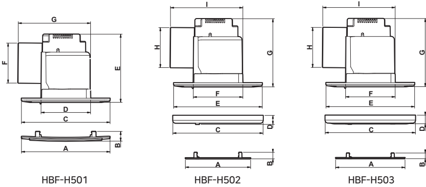
HBF-H501 제품 사이즈 (mm)
