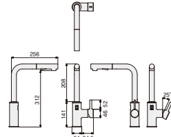
센서 수전 FC-YD1500SI_BN 타공 사이즈 : \phi 38mm
