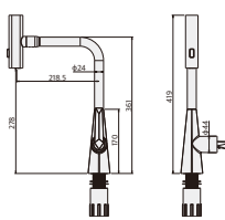
폰테302 FC-TB100 타공 사이즈 : \phi 33~35mm
