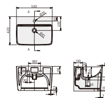
오브제 스퀘어 PB-192H 일체형 세면기 W530xL420xH360 L620
