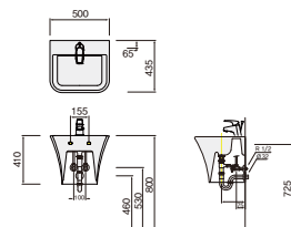
스퀘어벤트 PB-175H 일체형 세면기 W500×L435×H410 L620
