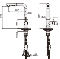
폰테 209 FC-LS100MS 타공 사이즈 : \phi 33~35mm
