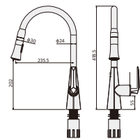
폰테301 FC-UB300 타공 사이즈 : \phi 33~35mm
