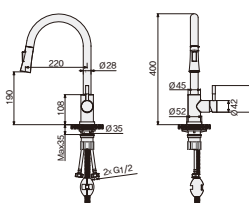
폰테 208 FC-US100MS 타공 사이즈 : \phi 33~35mm
