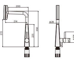
폰테206 FC-TS200 타공 사이즈 : \phi 33~35mm
