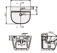
오브제 PB-168H 일체형 세면기 W520xL450xH370 L620
