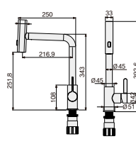
폰테 210 FC-TS100MS 타공 사이즈 : \phi 33~35mm
