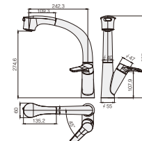
싱크 수전 FC-TB900 타공 사이즈 : \phi 36mm
