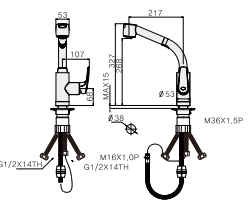
싱크 수전 FC-YA300 타공 사이즈 : \phi 38mm
