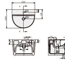
오브제 라운드 PB-167H 일체형 세면기 W530xL430xH360 L620
