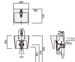
모던스퀘어 PB-132H 일체형 세면기 W460xL420xH380 L630
