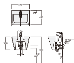
모던스퀘어 L PB-131H 일체형 세면기 W540xL435xH390 L620
