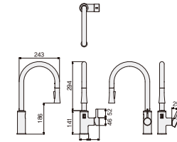
센서 수전 FC-YD1400SI_BN 타공 사이즈 : \phi 38mm
