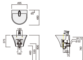
라운드벤트 PB-163H 일체형 세면기 W495×L480×H375 L630
