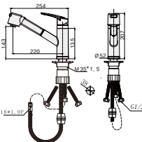
싱크 수전 FC-TA200 타공 사이즈 : \phi 38mm
