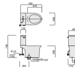
토네이도벤트 HZB-2000 투피스 양변기 W400×L700×H740
