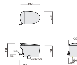
토네이도라운드 WB-10 원피스 양변기/직수형 W420×L660×H460
