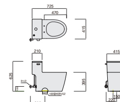
마제스틱 WB-600 원피스 양변기 W415×L725×H625
