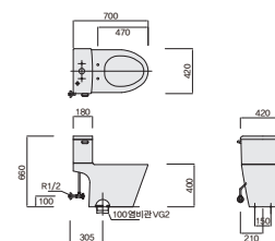
솔리드 HZB-3500 투피스 양변기 W420×L700×H660
