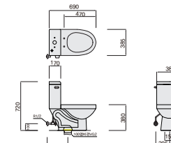
엔트리 HZB-7100/WB-7100 반피스 양변기 W385×L690×H720
