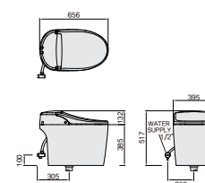
토네이도스마트 ALB-R14600 비데 일체형 양변기 / 직수형 W395×L656×H517
